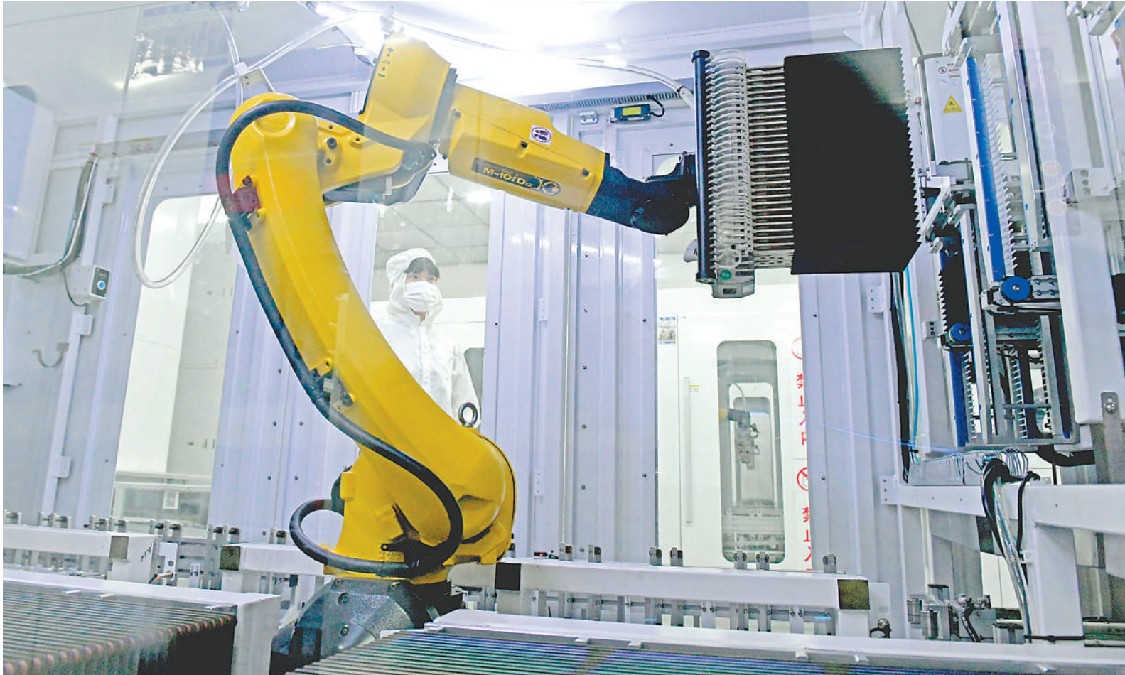
▲ 8月5日,位于淮南市凤台县的风台经济开发区,中环低碳(安徽)新能源光伏科技有限公司工人在生产N型TOPCon电池。 本报通讯员 陈彬 摄
